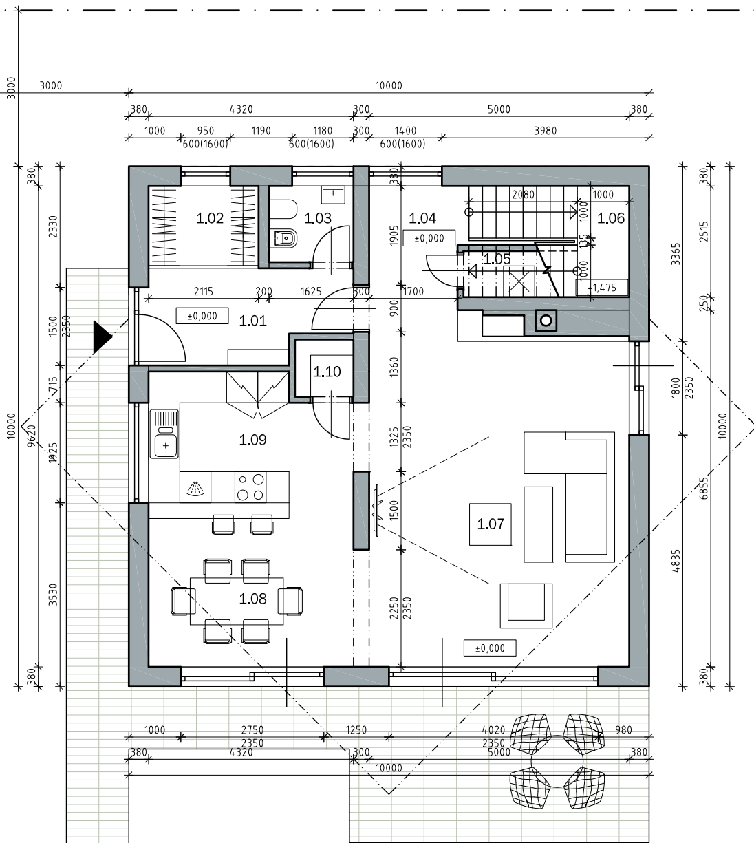
PÔDORYS 1.NP - PRÍZEMIE zastavaná plocha 100m 2
