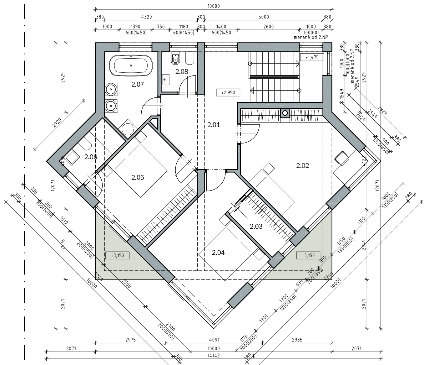
PÔDORYS 2.NP - POSCHODIE podlažná plocha 104m 2
